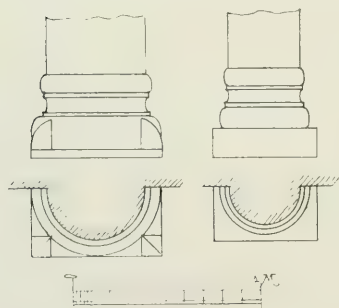
Fig. 40. Bazy słupów kryptowych.
